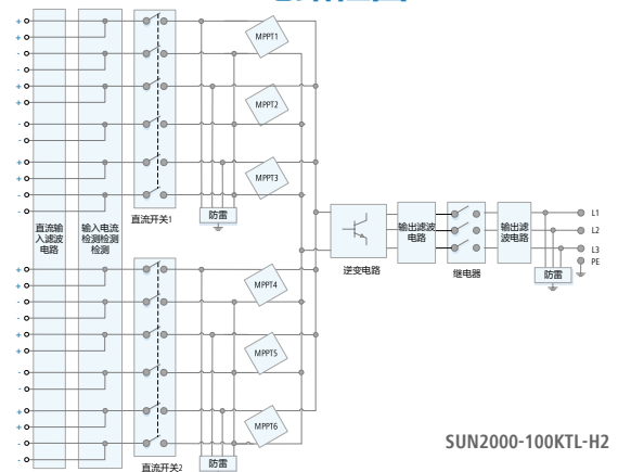
电路框图
