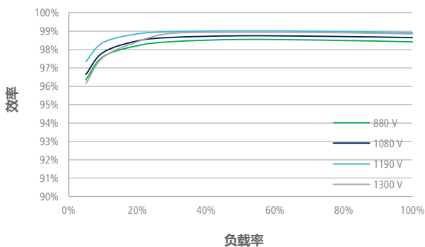
效率曲线
